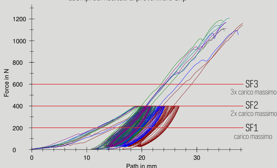
Esempi dei risultati di prova Micro Grip
